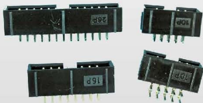
P/N:2170XXE(2.54mm) Dwg:2170-001
