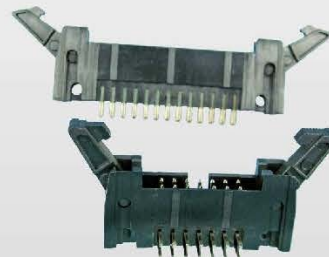
P/N:2171XXE(2.54mm) Dwg:2171-001
