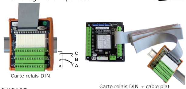
Carte relais DIN + câble plat
