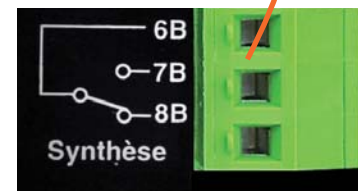
Sortie relais synthèse
