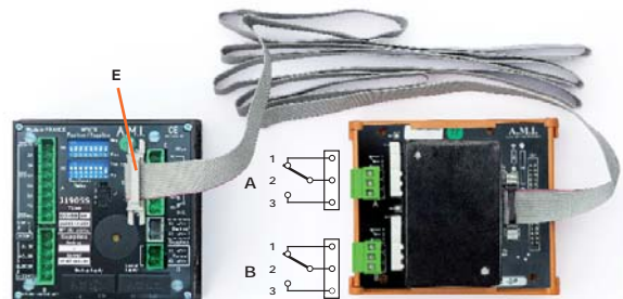
Carte M0901 «relais de report» type DIN connectée au panneau J1905S
